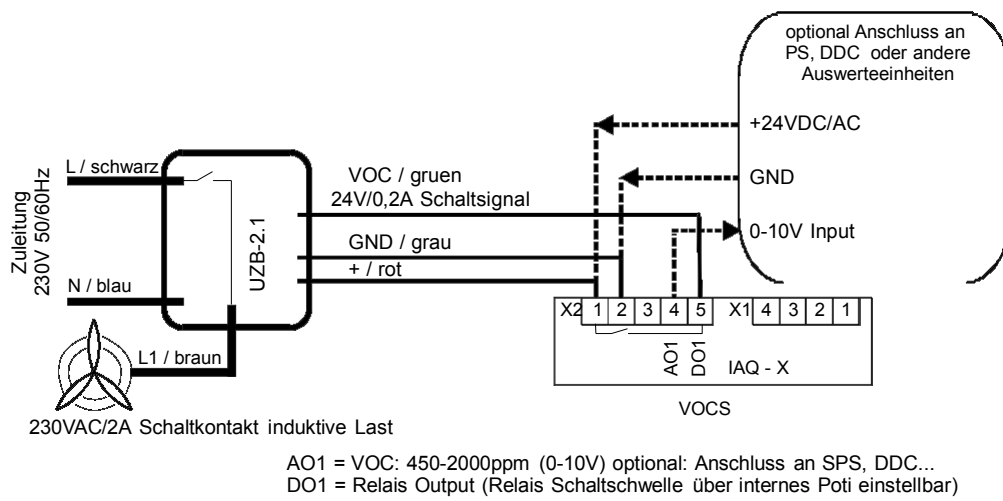
Abb. 9: Elektrischer Anschluss VOCS mit Netzteil UZB-2.11
